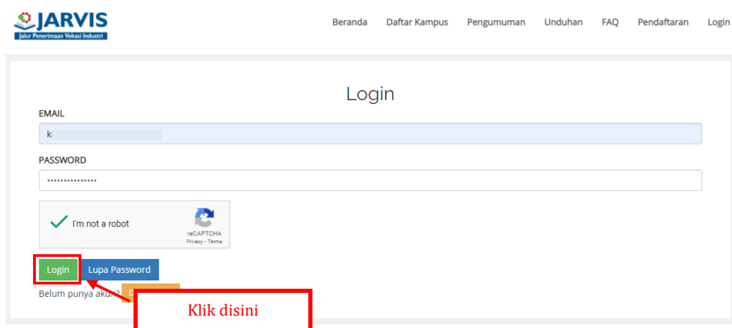
Gambar 6 Proses Login
